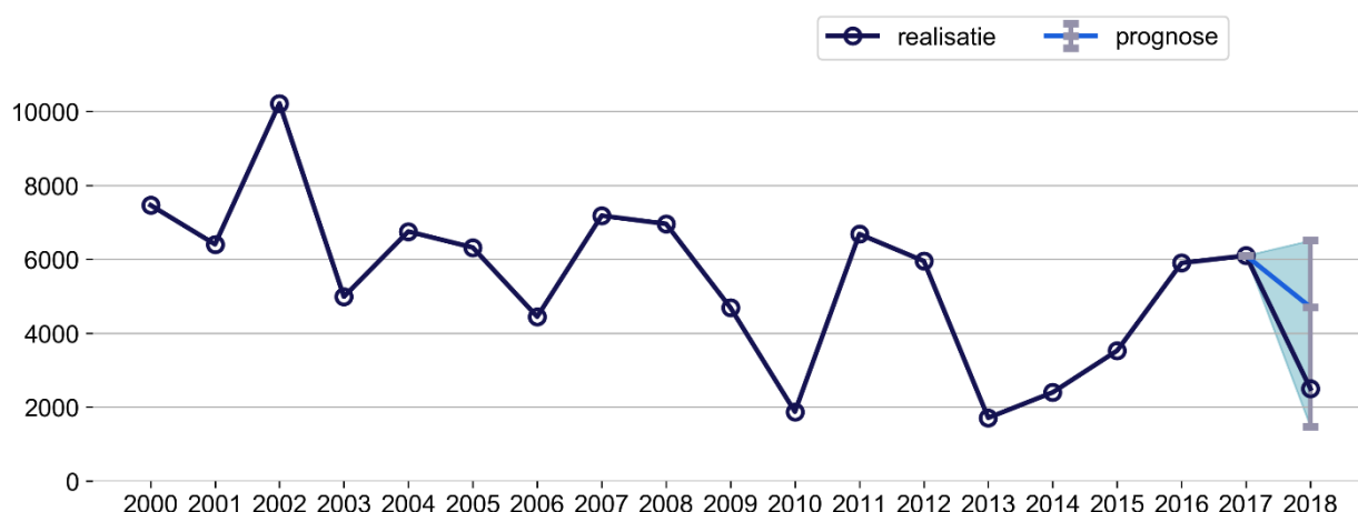
Figuur 6.3 Aantal woningen met een geluidbelasting van 48 dB(A) Lnight of meer, zonder meteomarge.
